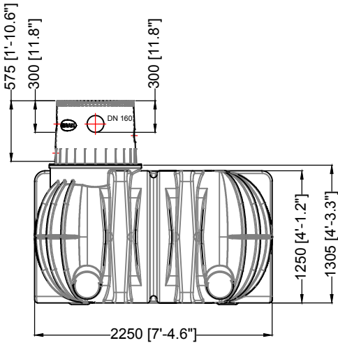
Ansicht A / View A
